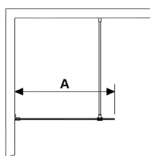
Skärmvägg fast
